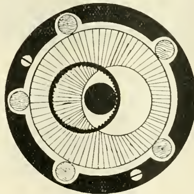
FIG. 2.—STUD EXTRACTOR.—L.V.R.R.
